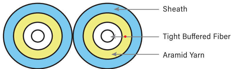
OM3 Cable
