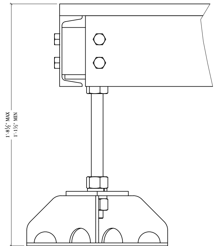
ELEVATION
